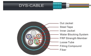
GYFTY53 Outdoor Cable
