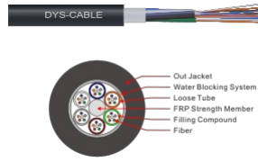
GYFTY Outdoor Cable
