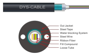
GYDXTW Outdoor Cable
